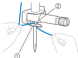
① Нитенаправитель игловодителя ② Язычок
