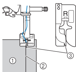
① Изнаночная сторона материала ② Складка по линии отгиба ③ Направляющая
