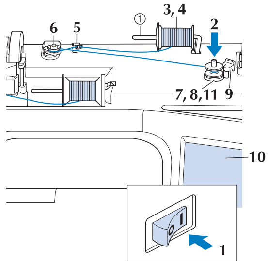
① Дополнительный стержень для установки катушки с нитью
